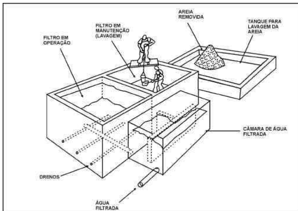
Figura 42 - Limpeza do Filtro Lento
