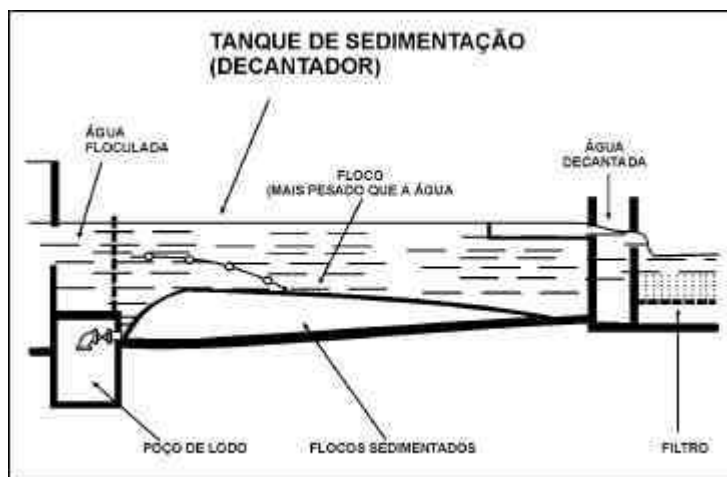
Figura 46 - Sedimentação
